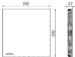
Рисунок 1 Светильник «L-office 32 S Premium»
