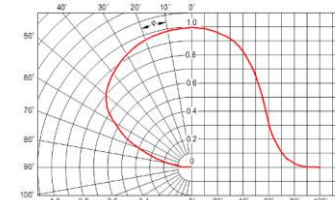
Рисунок 5 Типы КСС
