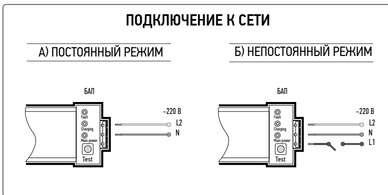
PWP-C3-E1 1200 (с БАП)
