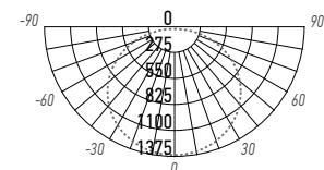
PPL PRO 6060 40W
