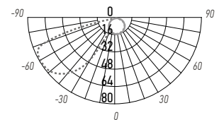
PST/W R150 2W
