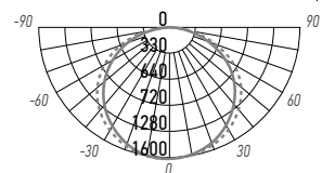
PPL PRO-3 36W PRISMA
