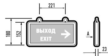
PEL 102-2 3W 1.2V IP20 "ВЫХОД-EXIT" / СТРЕЛКА НАПРАВЛЕНИЯ
