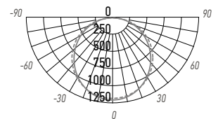
PWP-C5 PRO 36W
