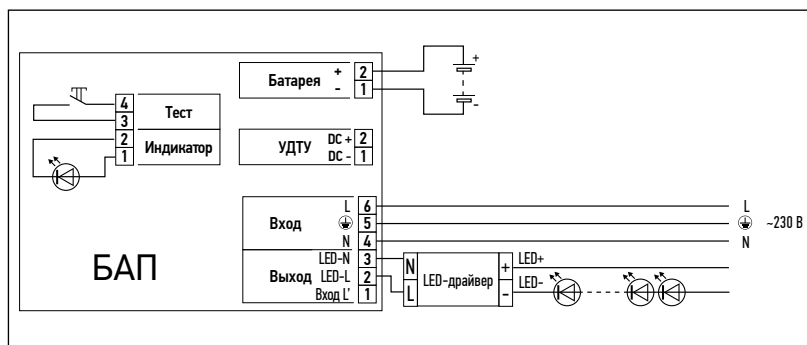
Режимы работы БАП: Непостоянный режим
