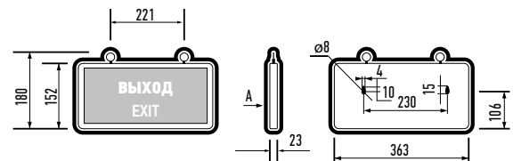
PEL 101-1 3W 1.2V IP20 "ВЫХОД-EXIT"
