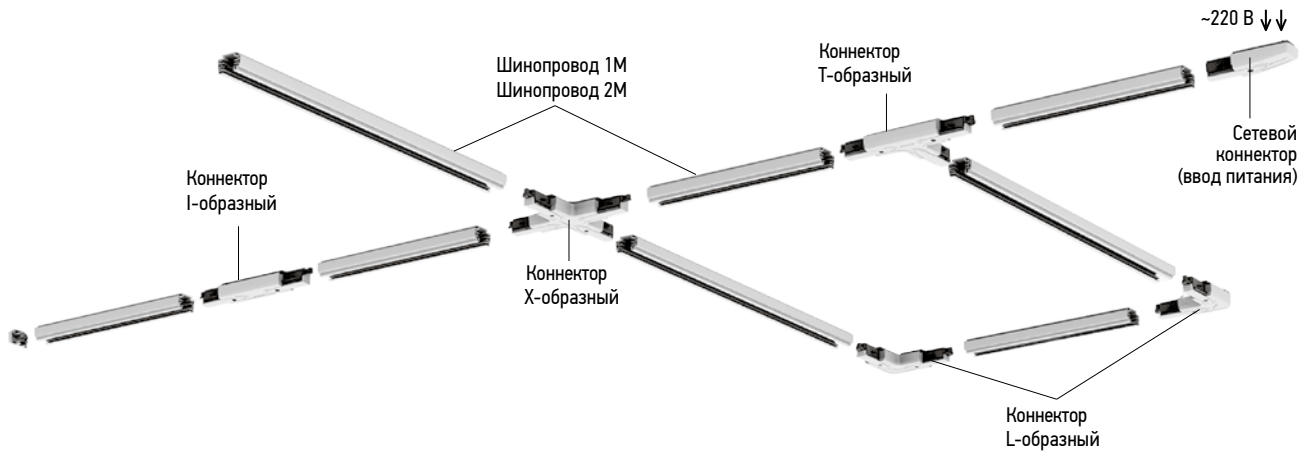
СХЕМА НАКЛАДНОГО МОНТАЖА
