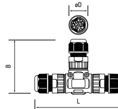
PCC-T3-F 3x2.5 24A IP68
