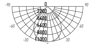
PHB 04 PRO-5 150W
