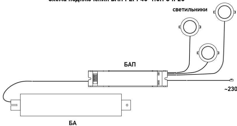
Схема подключения БАП РЕРР40-1.0Н U IP20
