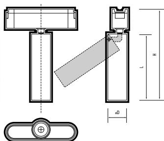
MTR16 2112 12W 3000K BL 24° IP40
