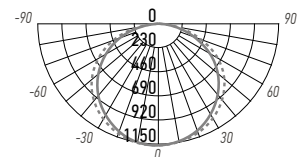
PPL SPEC 1 36W OP
