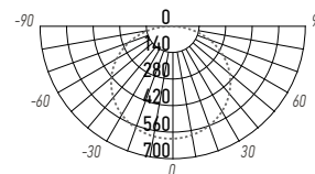
РРО-03 600/К 20W
