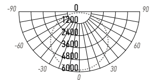
PHB UFO 04 150W
