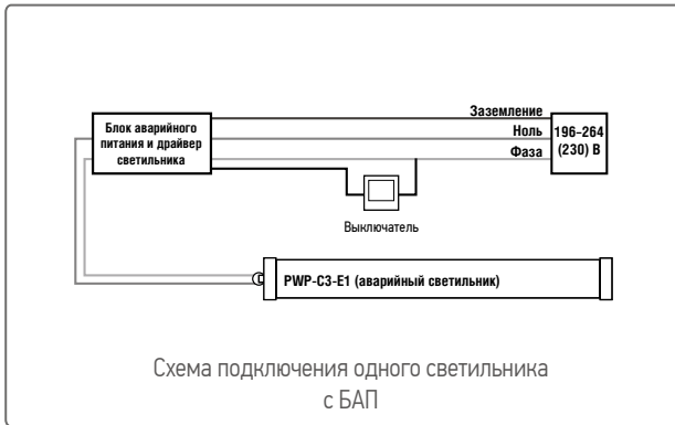
PWP-C3-E1 1500 (с БАП)
