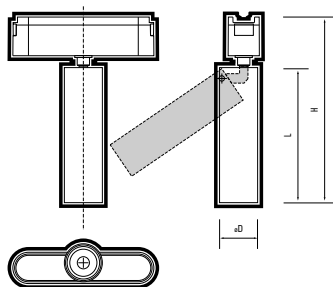
MTR16 2008 8W BL 24° IP20
