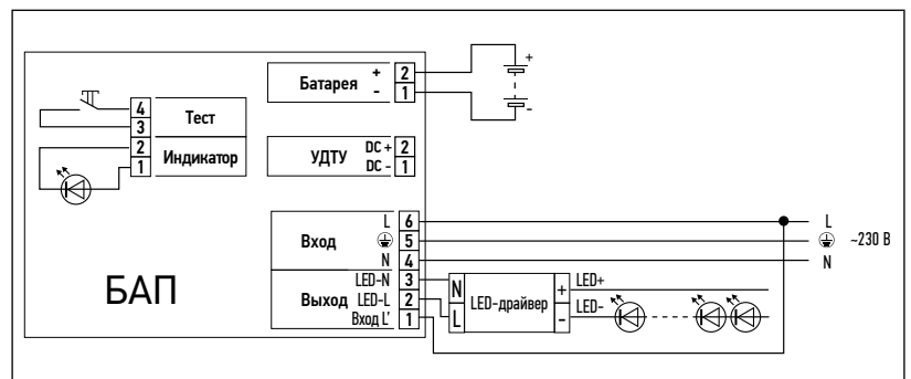
Режимы работы БАП: Постоянный режим
