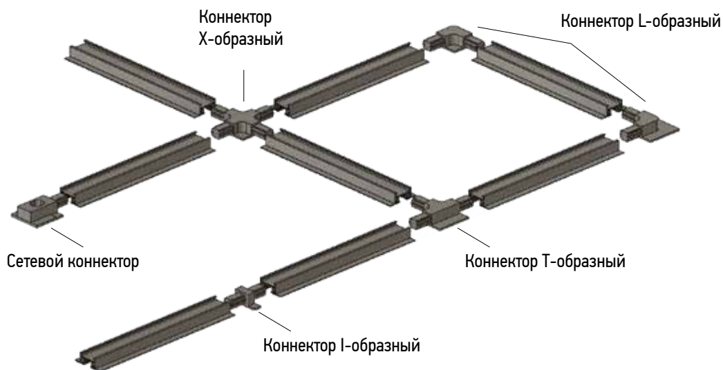
СХЕМА ВСТРАИВАЕМОГО МОНТАЖА
