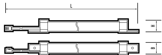
PEPP40-1.0H IP20. (Габаритные размеры)
