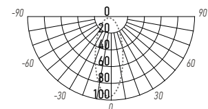
PWW 1000 24V SNAKE (ОДНОГО МОДУЛЯ)
