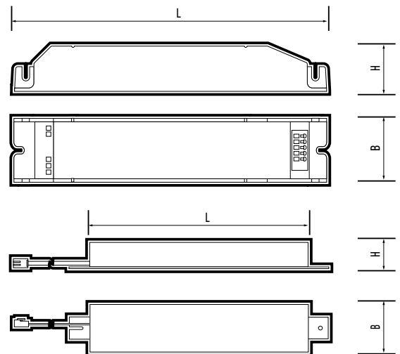
РЕРР40-1.0Н U IP20
