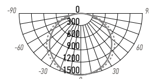
PPL 588/G 36W PRISMA
