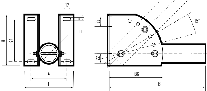
ДЕРЖАТЕЛЬ НА СТЕНУ ДЛЯ PSL D40*1.5
