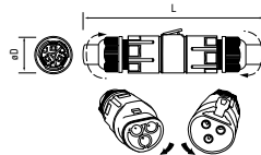
PCC-I3-FD 3x2.5 24A IP68
