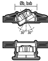
Схема установки PSP-R
