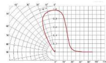
Исполнение «Г60»
